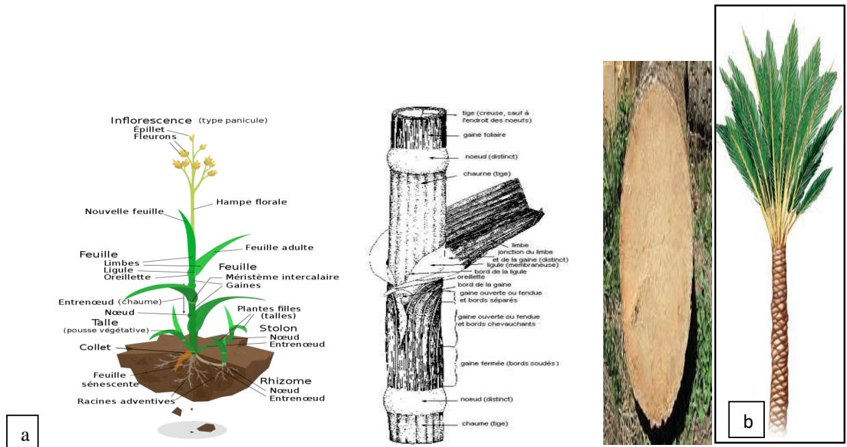
Figure 15: Tige de graminée (chaume) (a) et tronc d'un palmier (stipe) (b).
