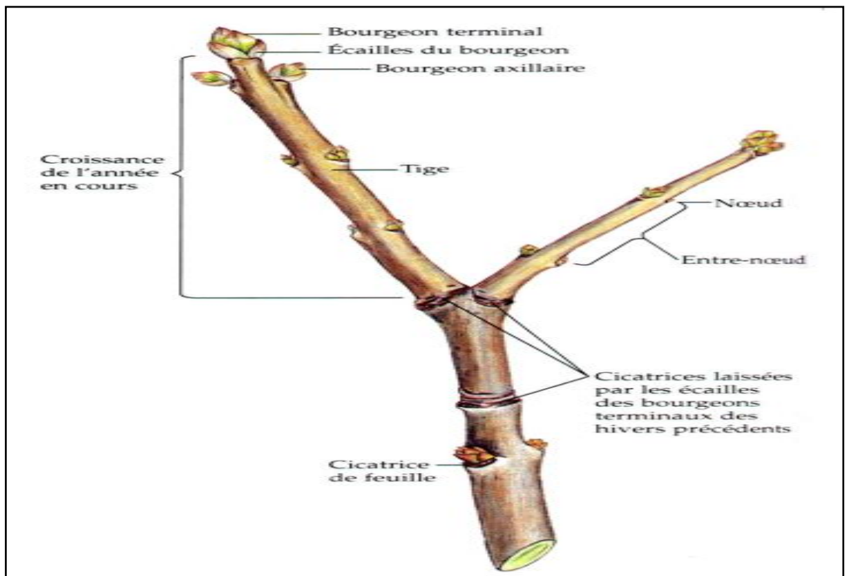
Figure 3 : Morphologie générale d'une tige herbacée
