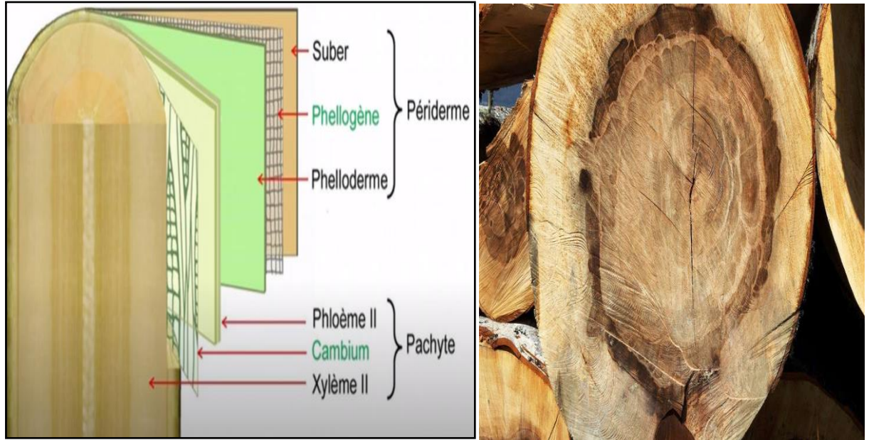
Figure 10 : Structure secondaire (Formation du bois, Cernes de croissance, cœur et aubier du bois)
