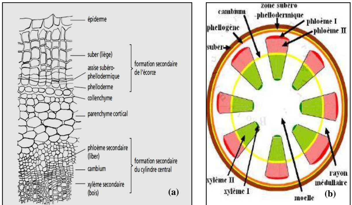
Figure 8 : Schéma d'une coupe transversale d'une tige âgée (a) ; Coupe entière (1:cambium interfasciculaire 2: cambium intrafasciculaire) (b)
