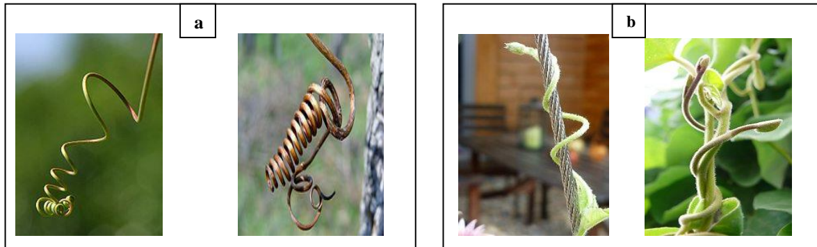
Vrille de vigne, en croissance Vrille de vigne, lignifiée.
