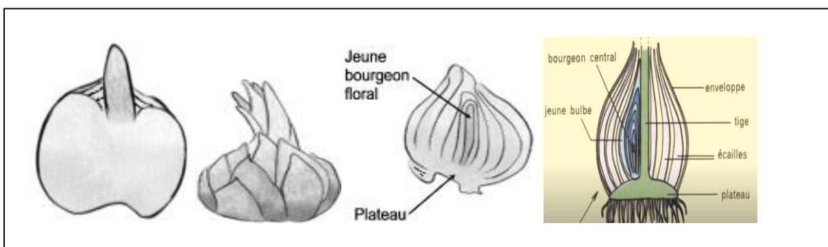
Figure 24 : Section longitudinale d'un bulbe solide de Crocus ; Bulbe écailleux du Lis ; Section longitudinale d'un bulbe tunique de Tulipe
