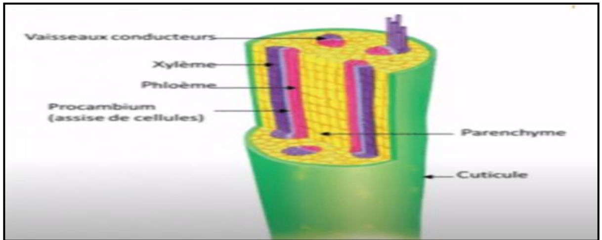
Figure 4 : Disposition des tissus conducteurs au niveau de la tige
