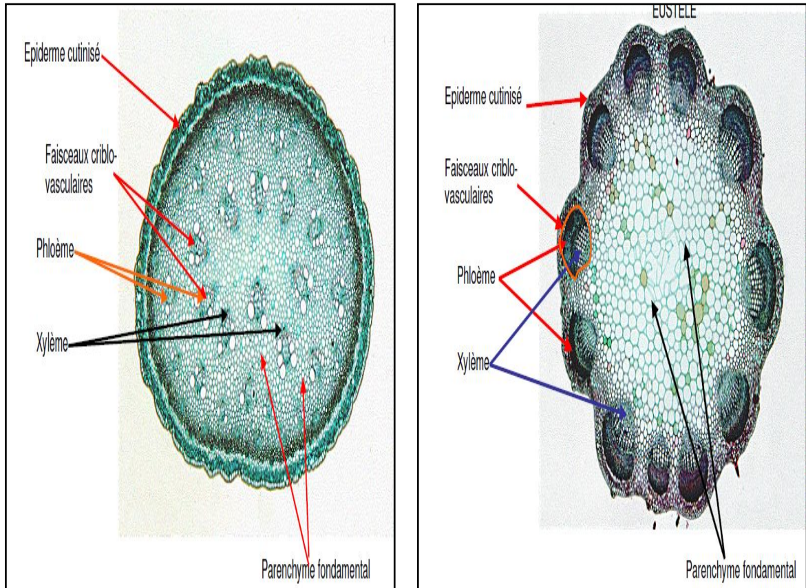
Figure 14 : Coupe transversale de la tige d'asperge (monocotylédone) et de trèfle (dicotylédone)
