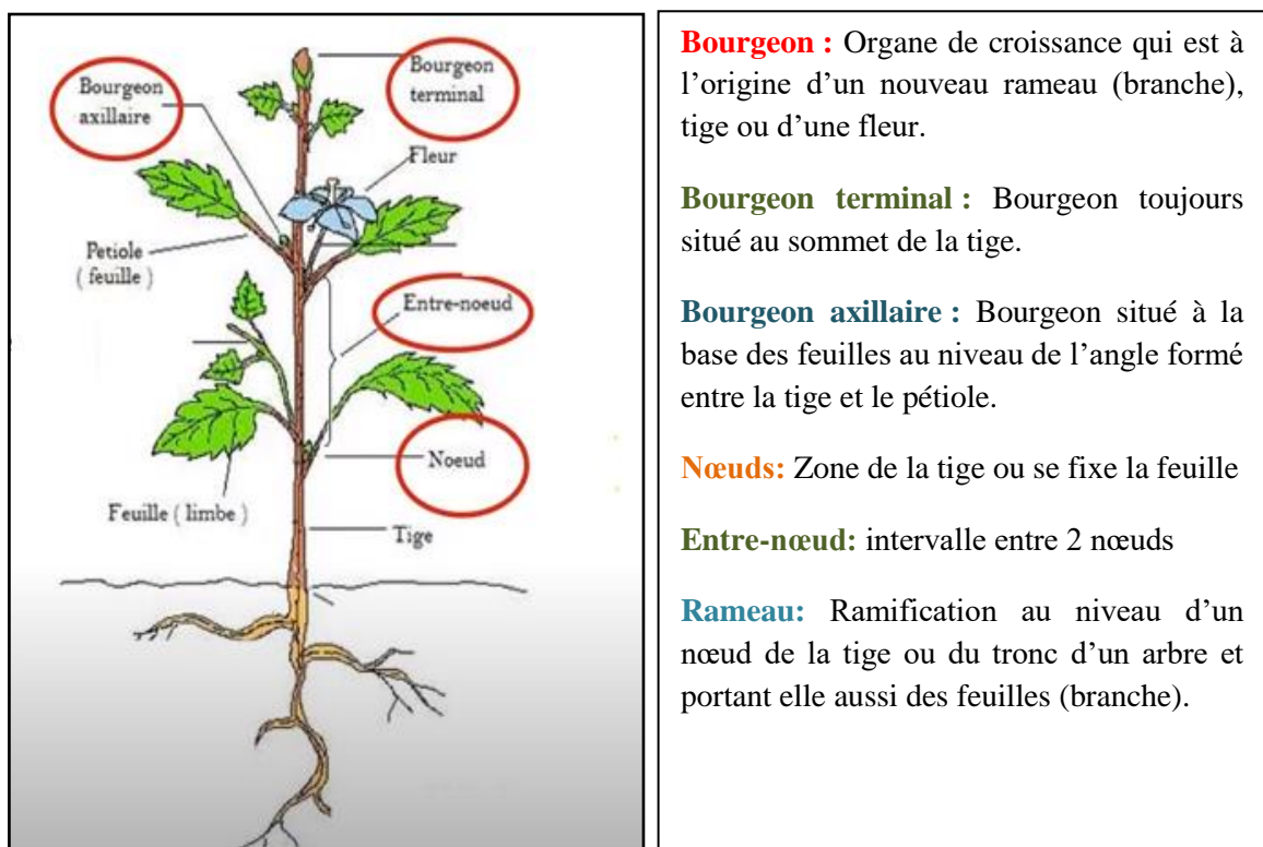
Figure 1 : Emplacement des bourgeons et des nœuds au niveau de la tige
