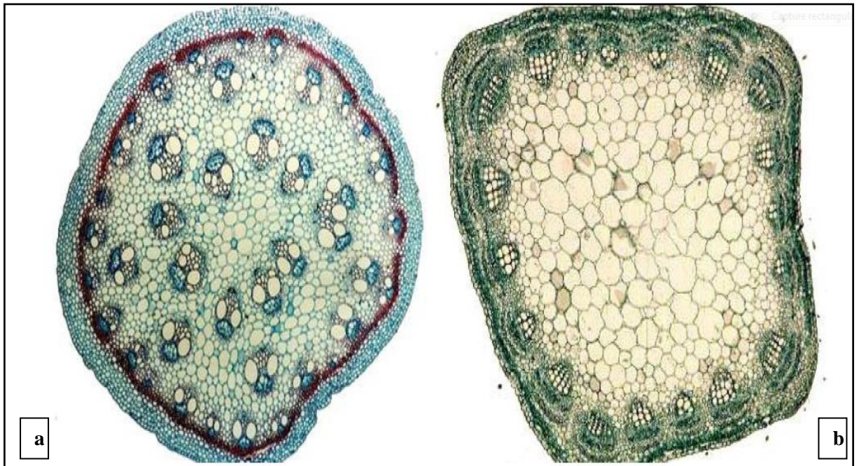
Figure 13 : Coupe transversale d'une tige et monocotylédone (a) dicotylédone (b)
