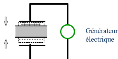
2-Effet Piézoélectrique inverse (émission)
