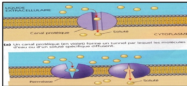
Figure.3: Récepteur protéine de transport
