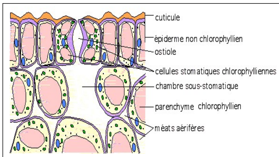
Figure 12 : Cellules épidermiques
