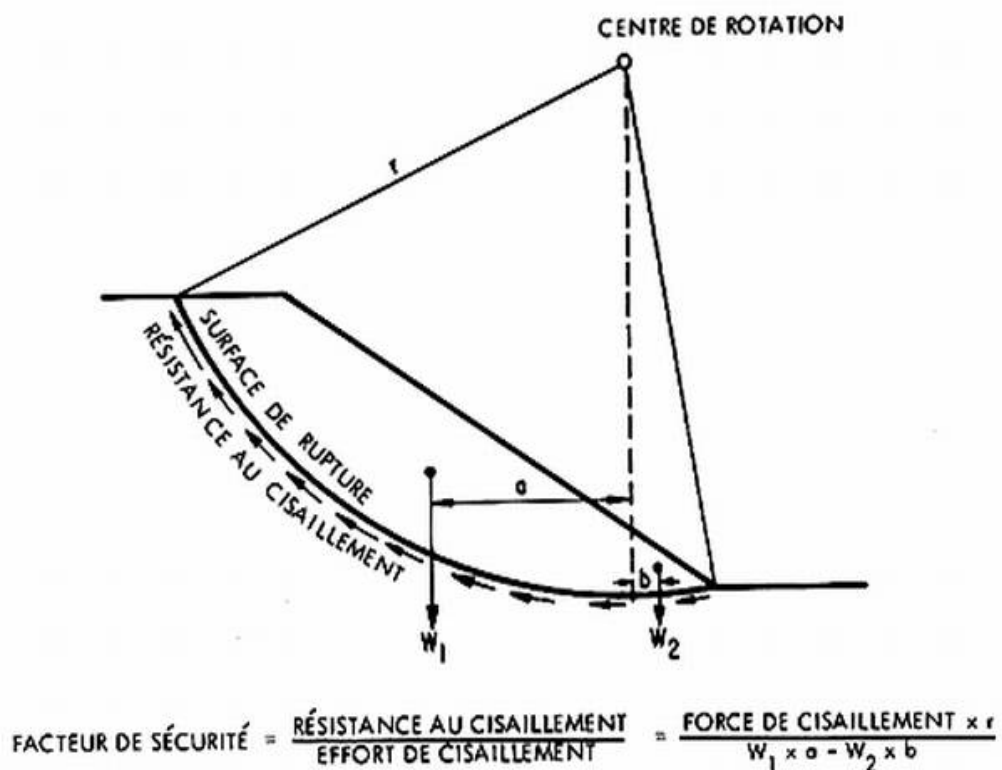
Fig. 30 : Le facteur de sécurité d'un glissement
